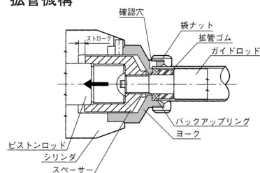
拡管機構
